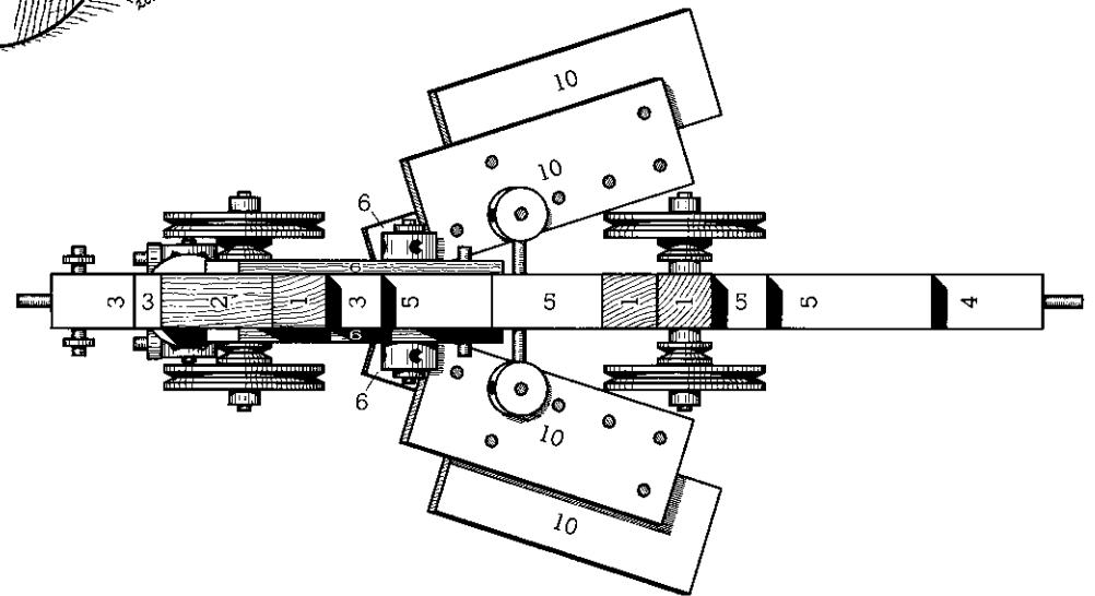
282/3 Ansicht von unten | Bottom view | Vue de dessous
