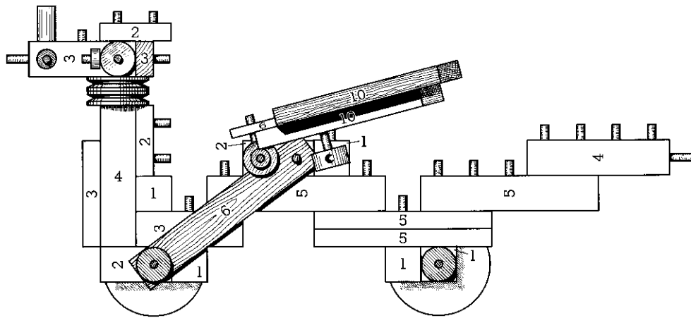
282/2 Ansicht von der Seite | Side view | Vue de côté
