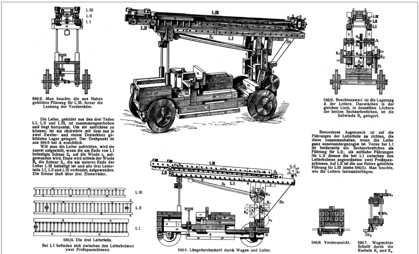
Bauanleitung Nummer 586 erläutert den Bau einer dreiteiligen Feuerwehrlleiter und war dem Baukasten Nr. 6 beige packt
